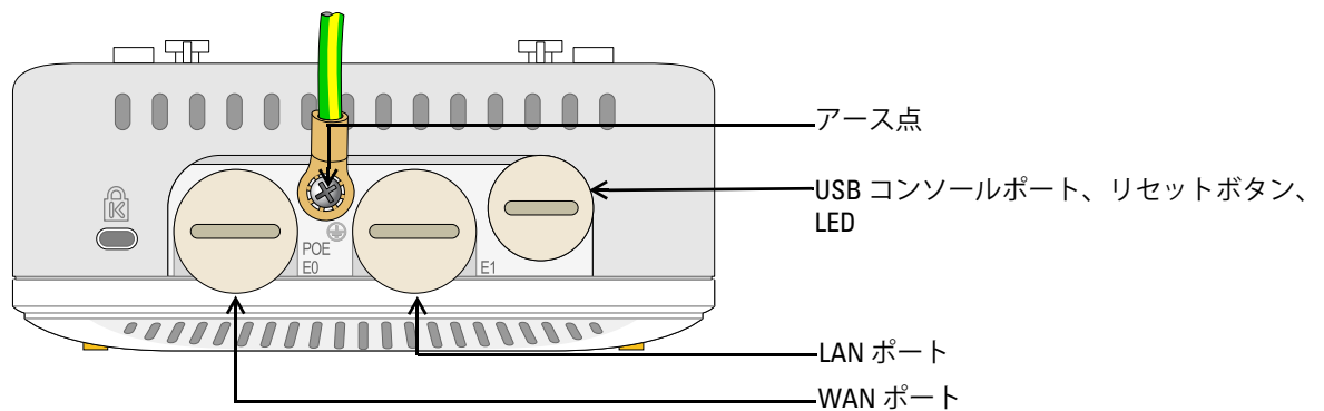
図 2 W-AP228 の底面
