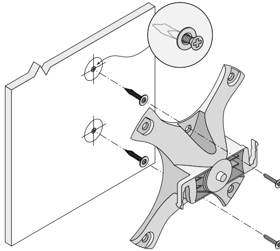
図6 アダプタを壁に取り付ける (代替方法)
