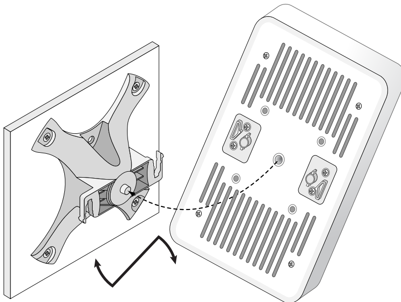
図7 マウント用ブラケットへの AP の取り付け
