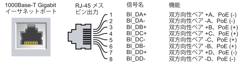
図3 Gigabit イーサネットポートピン出力
