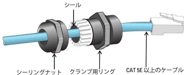
図 9 ケーブルグランドの取り付け
